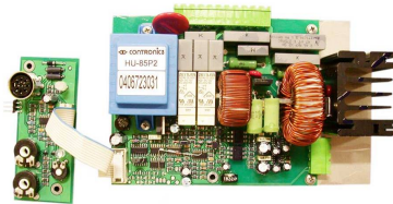
Typ HP HU-85P2 Hauptplatine zu HU 85
